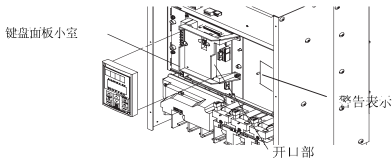
图 1-3-4 卸下键盘面板 ( \geq 30\text{kW} )
