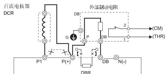
图 2-3-4 连接图
