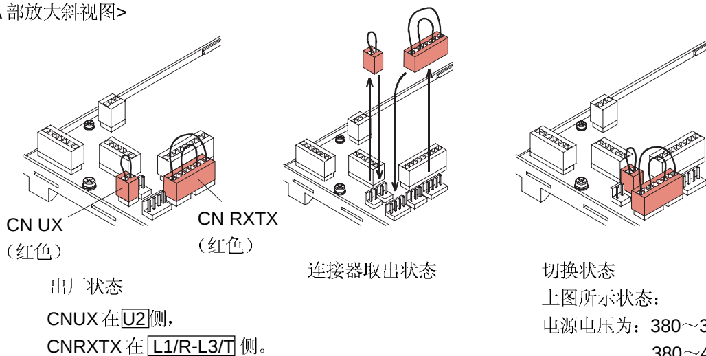
图 2-3-8 电源切换连接器 (≥ 30kW 变频器)
